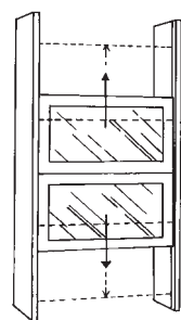
Elemento alto saliscendi da 90 con vetro acidato.
