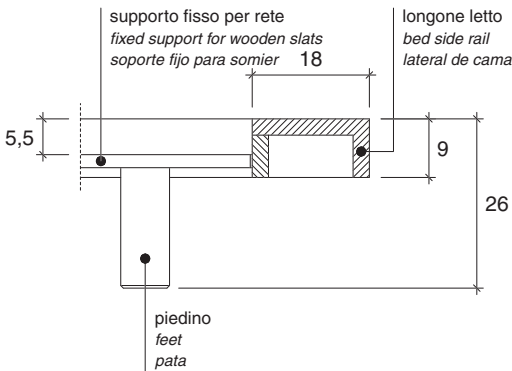
Posizionamento fisso del supporto rete, per letti con piedi Fixed positioning of wooden slats support for beds with feet Colocación fija de soporte de somier para cama con patas
