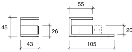
C105 con 1 comodino C105 with 1 night table C105 con 1 mesita de noche
