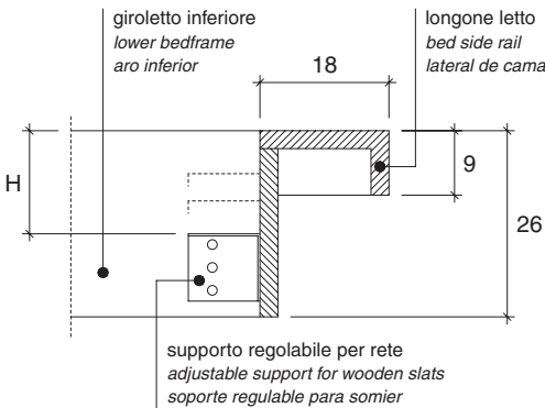
Posizionamento regolabile del supporto rete, per letti con box fisso Adjustable positioning of wooden slats support for beds with fixed box Colocación regulable de soporte de somier para camas con box fijo H = 6 - 8 - 9,2 - 11,2 - 14,4
