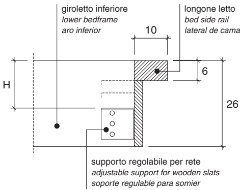
Posizionamento regolabile del supporto rete, per letti con box fisso Adjustable positioning of wooden slats support for beds with fixed box Colocación regulable de soporte de somier para camas con box fijo H = 6,6 - 8,2 - 11,4 - 14,6
