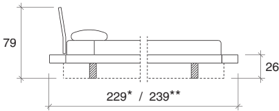
Testiera tipo "A" Headboard mod. "A" Cabezal tipo "A"
