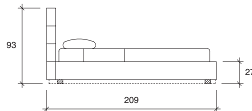
letto per rete e materasso larghi 150 e profondi 190 Bed for 150 cm wide and 190 cm deep wooden slats and mattress Cama para somier y colchón de ancho 150 cm y fondo 190 cm
