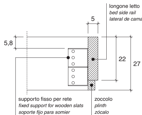
Posizionamento regolabile del supporto rete, per letti con box fisso Adjustable positioning of wooden slats support for beds with fixed box Colocación regulable de soporte de somier para camas con box fijo
