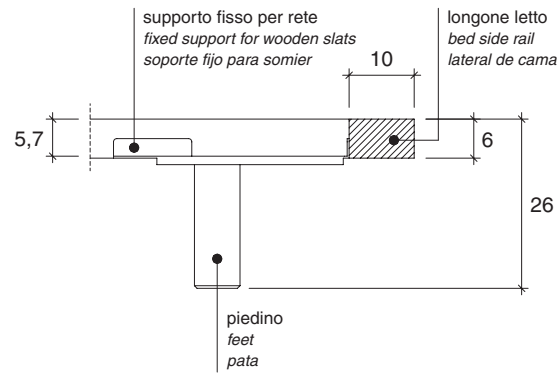
Posizionamento fisso del supporto rete, per letti con piedi Fixed positioning of wooden slats support for beds with feet Colocación fija de soporte de somier para cama con patas
