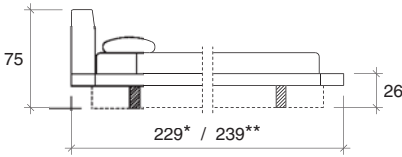
Testiera tipo "C" Headboard mod. "C" Cabezal tipo "C"
