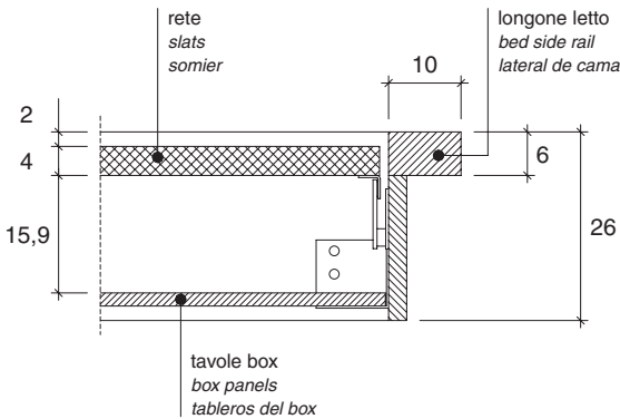
Posizionamento rete per letti con box apribile Positioning of wooden slats for storage beds Colocación de somier para camas abatibles
