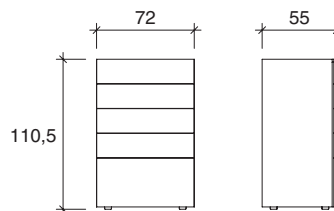
Settimino Tall boy Cómoda
