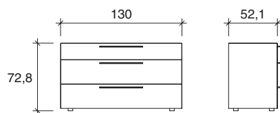
Comò Chest of drawers Cómoda
