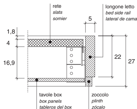
Posizionamento rete per letti con box apribile Positioning of wooden slats for storage beds Colocación de somier para camas abatibles
