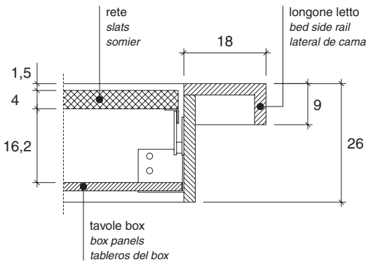
Posizionamento rete per letti con box apribile Positioning of wooden slats for storage beds Colocación de somier para camas abatibles
