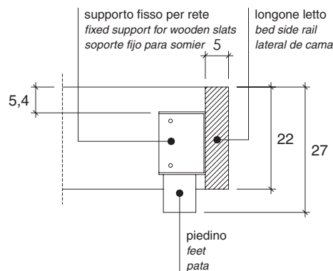
Posizionamento fisso del supporto rete, per letti con piedi Fixed positioning of wooden slats support for beds with feet Colocación fija de soporte de somier para cama con patas
